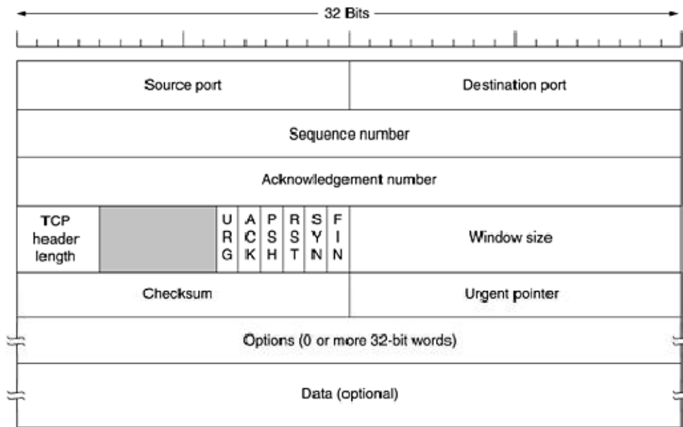
TCP HEADER
