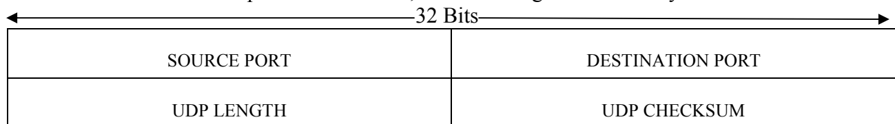
UDP HEADER
